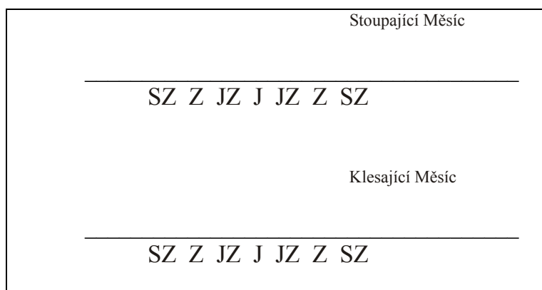
siderický Měsíc (stoupající - klesající)
